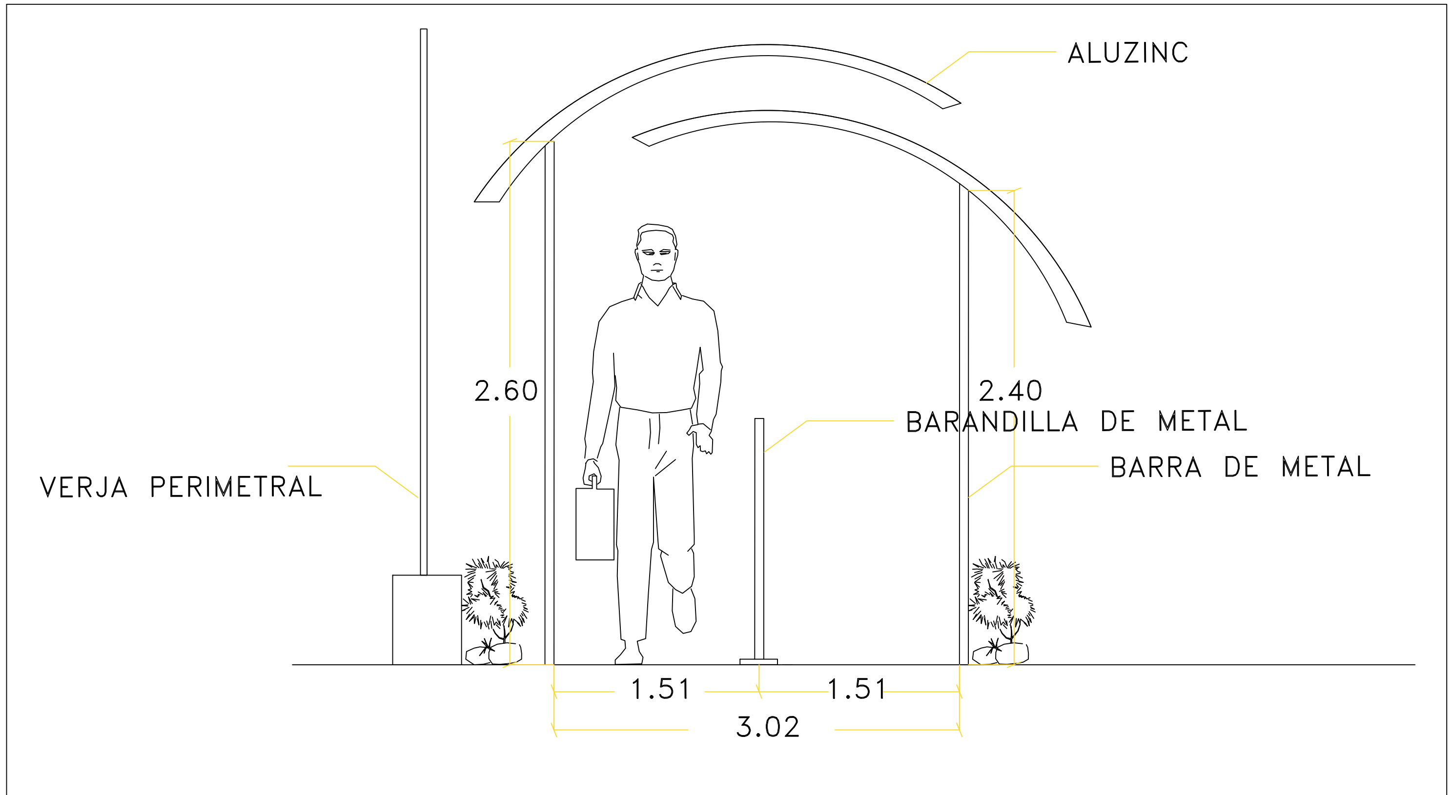
DETALLE DE ESTRUCTURA PEATONAL
